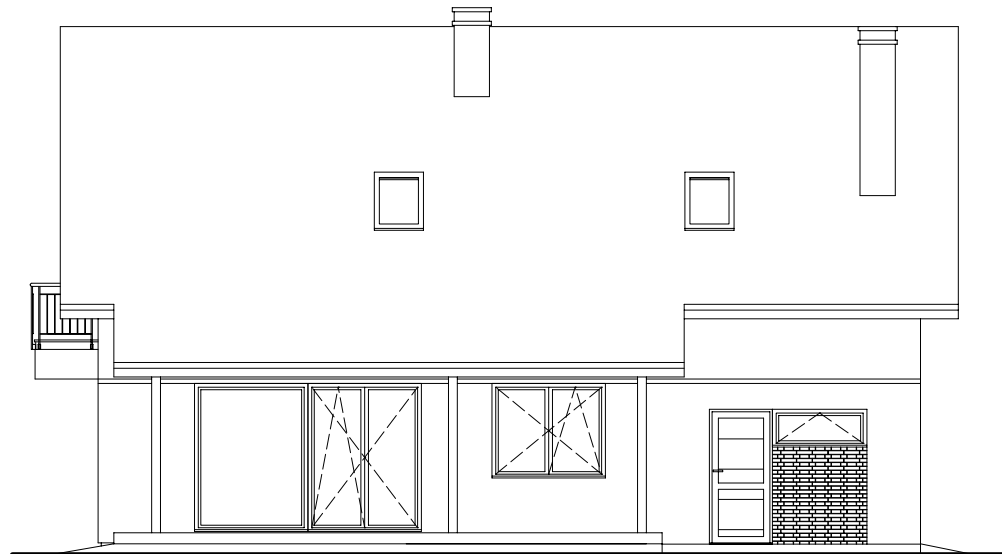
ELEWACJA OGRODOWA
